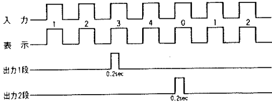
カウンタ2段プリセット加算 (瞬時リセット動作、1段目・2段目ワンショット出力)
