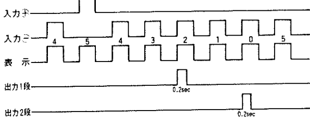
カウンタ2段プリセット加減算 (瞬時リセット動作、1段目・2段目ワンショット出力、書き込み)
