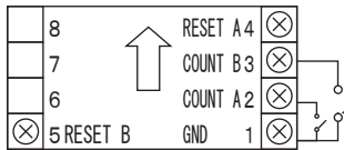
加算入力(有接点、オープンコレクタ入力) G37-101
