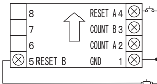
リセット入力 G37-101・102
