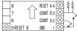
加算入力(有接点電圧入力) G37-102
