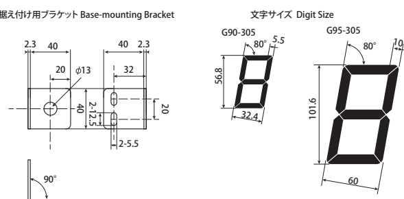
据え付け用ブラケット Base-mounting Bracket
